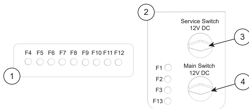
Abbildung 8.1 Yamarin 63 DC/BR Hauptschalter und Sicherungspanel
