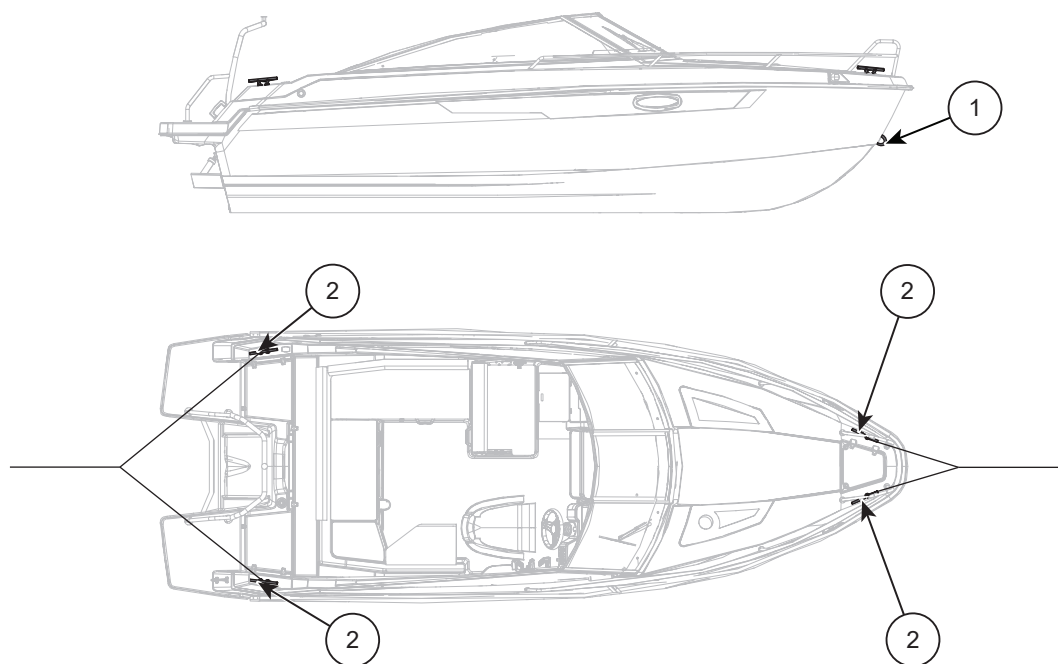
Abbildung 5.7 Yamarin 63 DC Befestigungs- und Schlepppunkte
