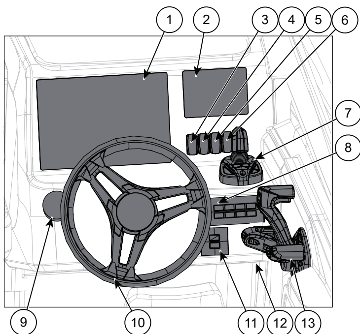
Abbildung 5.1 Yamarin 63 DC/BR Bedienelemente am Steuerstand
