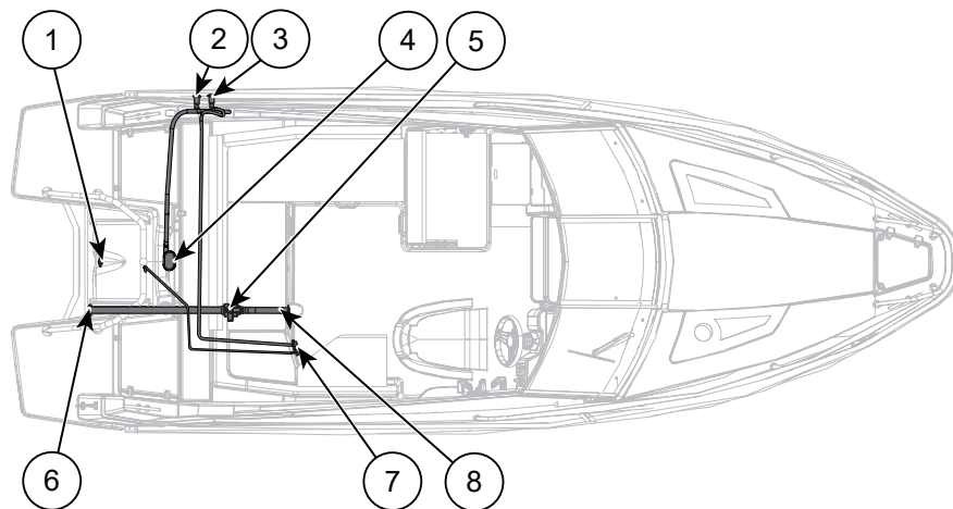
Abbildung 9.1 Yamarin 63 DC Bilgenpumpen und Entwässerung
