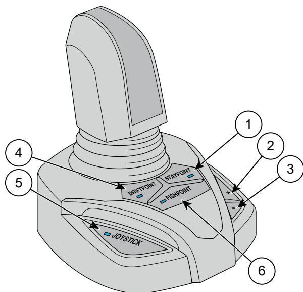
Abbildung 5.4 Joystick und Funktionstasten
