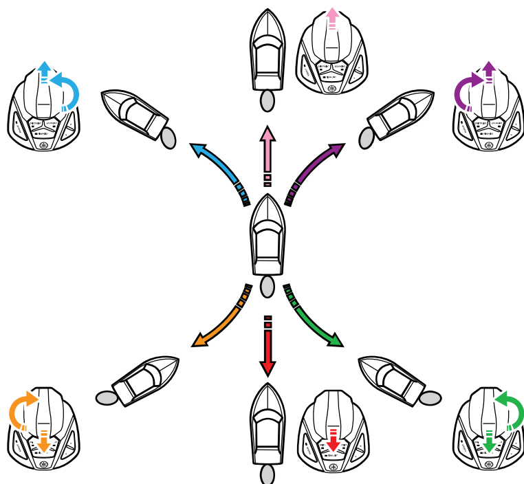
Abbildung 5.5 Joystick-Betrieb mit einem einmotorigen Boot
