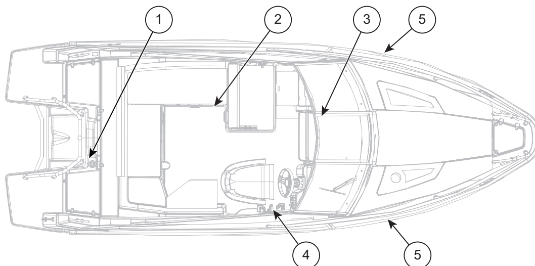
Abbildung 2.1 Yamarin 63 DC Sicherheitsetiketten.
