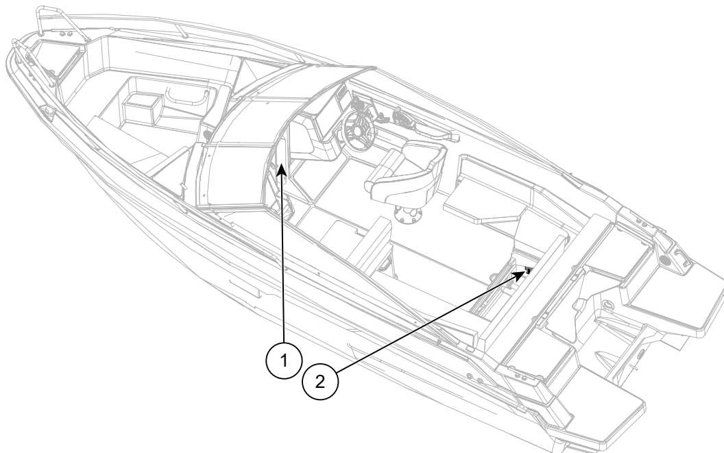
Abbildung 8.3 Yamarin 63 BR Sicherungspanel
